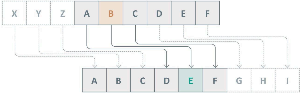
شكل 3.7: تمثيل خوارزمية تشفير قيصر باستخدام مفتاح = 3
