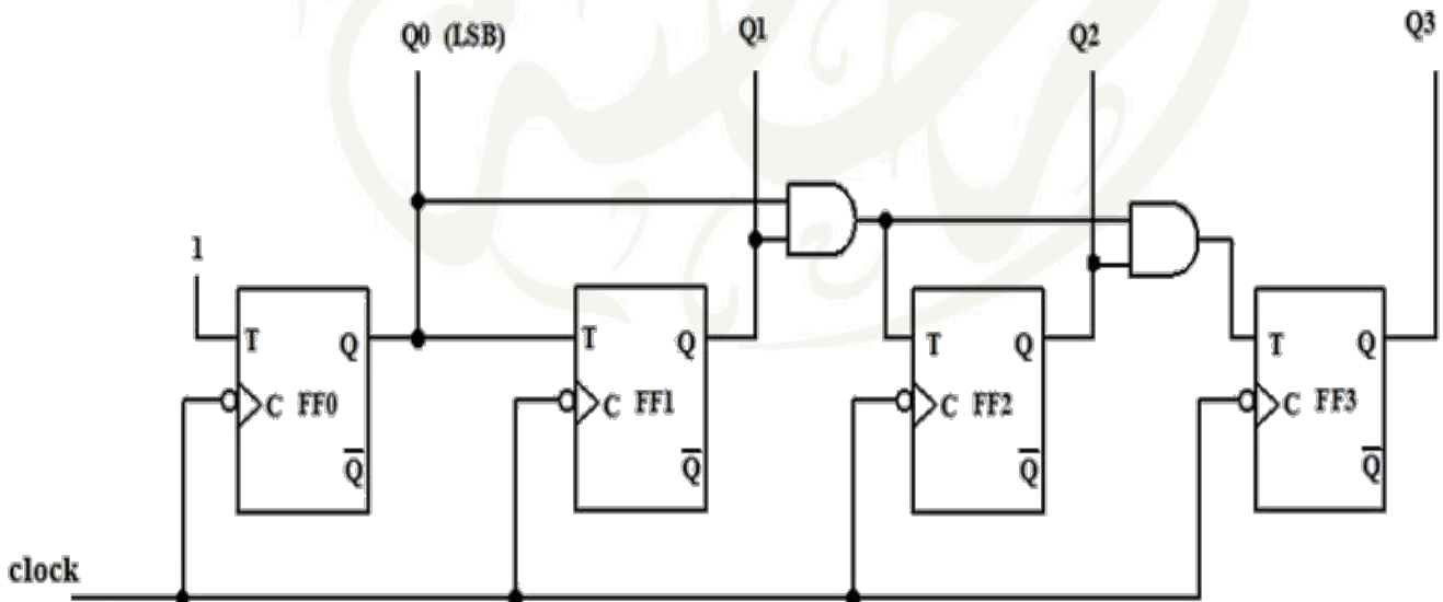
هذا العداد يعد من ٠ إلى ١٥
