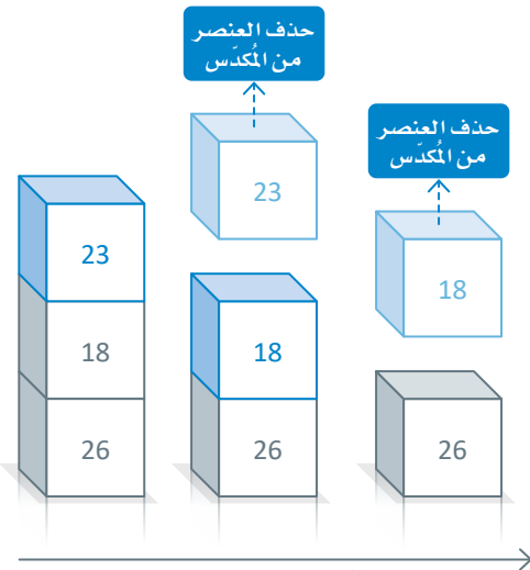
شكل 1.21: حذف العناصر
