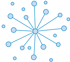
شكل 3.16: تمثيل عنقود
