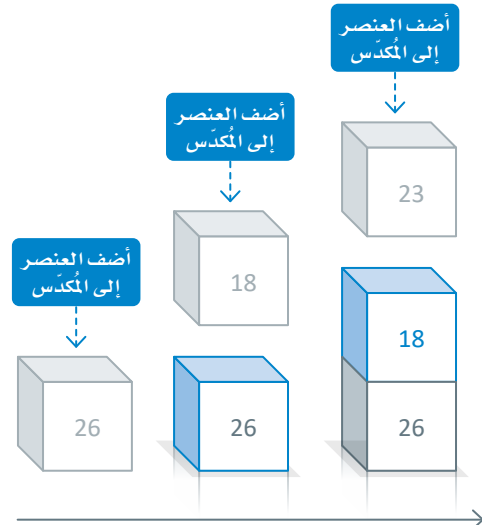
شكل 1.20: إضافة العناصر
